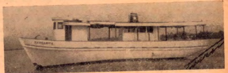
LANCHA MARGARITA ya fuera del astillero. — Quilla 30 pies; Eslora 45 pies; Manga 11 pies; Puntal 5 pies. — —Reconstruida en 1950.
